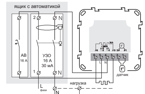
Схема 2. Подключение автоматического выключателя и УЗО
