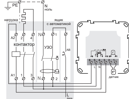
Схема 3. Подключение через контактор
